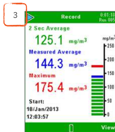
Mesure et enregistrement
